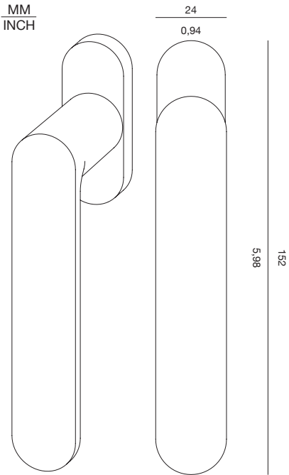
QUADRO / SPINDLE 7 MM / 0,27 INCH
