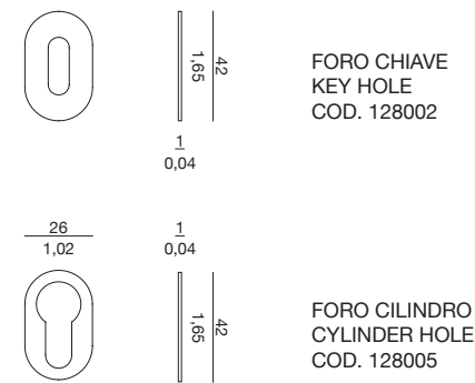
A. BOCCHETTA SLIM / SLIM ESCUTCHEON
