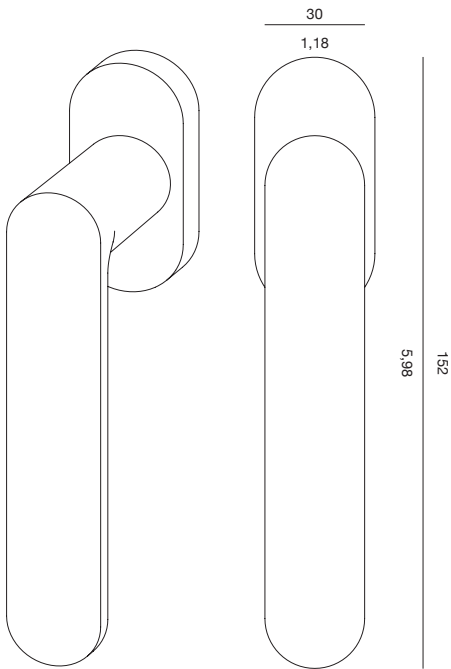
QUADRO / SPINDLE 7 MM / 0,27 INCH
